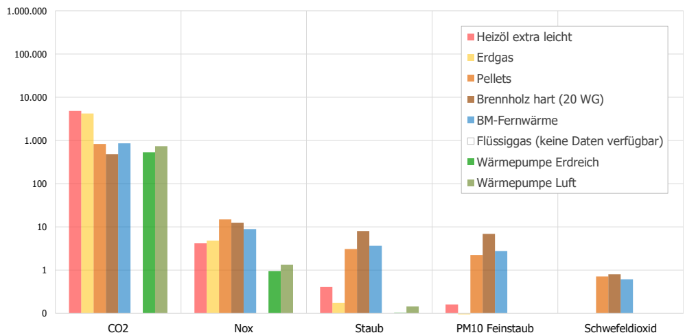
Quelle: Umweltbundesamt 2014 - Emissionsfaktoren unterschiedlicher Heizsysteme
